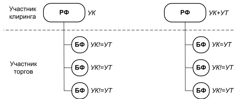
Рис. 2. Иерархия сущностей
