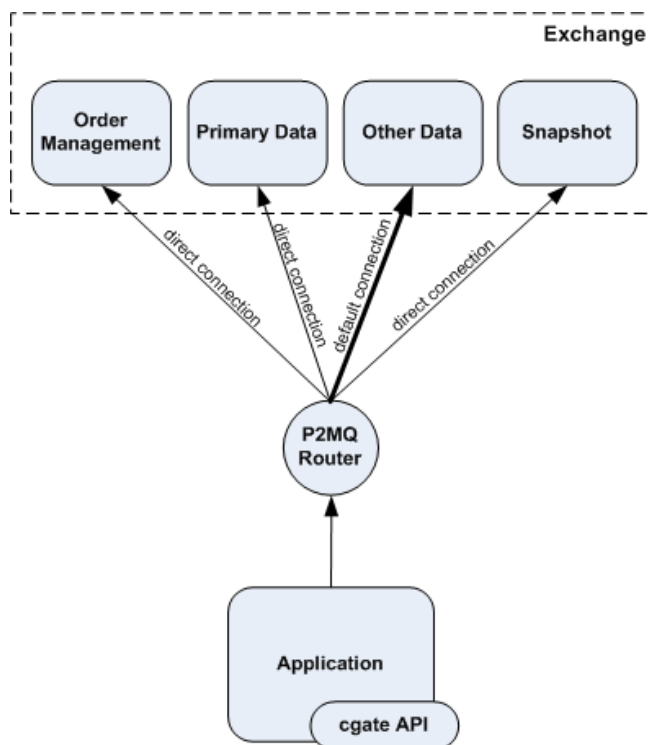
Рис. 7. Шлюз SPECTRA Plaza-2. Архитектура
